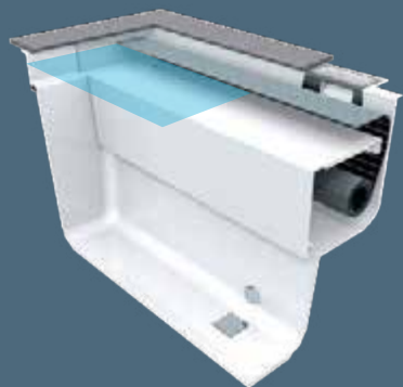
Der Rollladenschacht verlängert das Becken um 50 cm.
